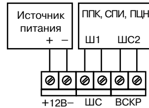
Рисунок 2 – Схема подключения извещателя с отдельными шлейфами сигнализации и вскрытия корпуса
